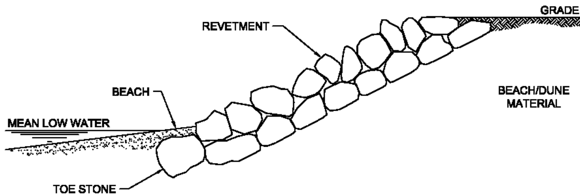
REVETMENT
